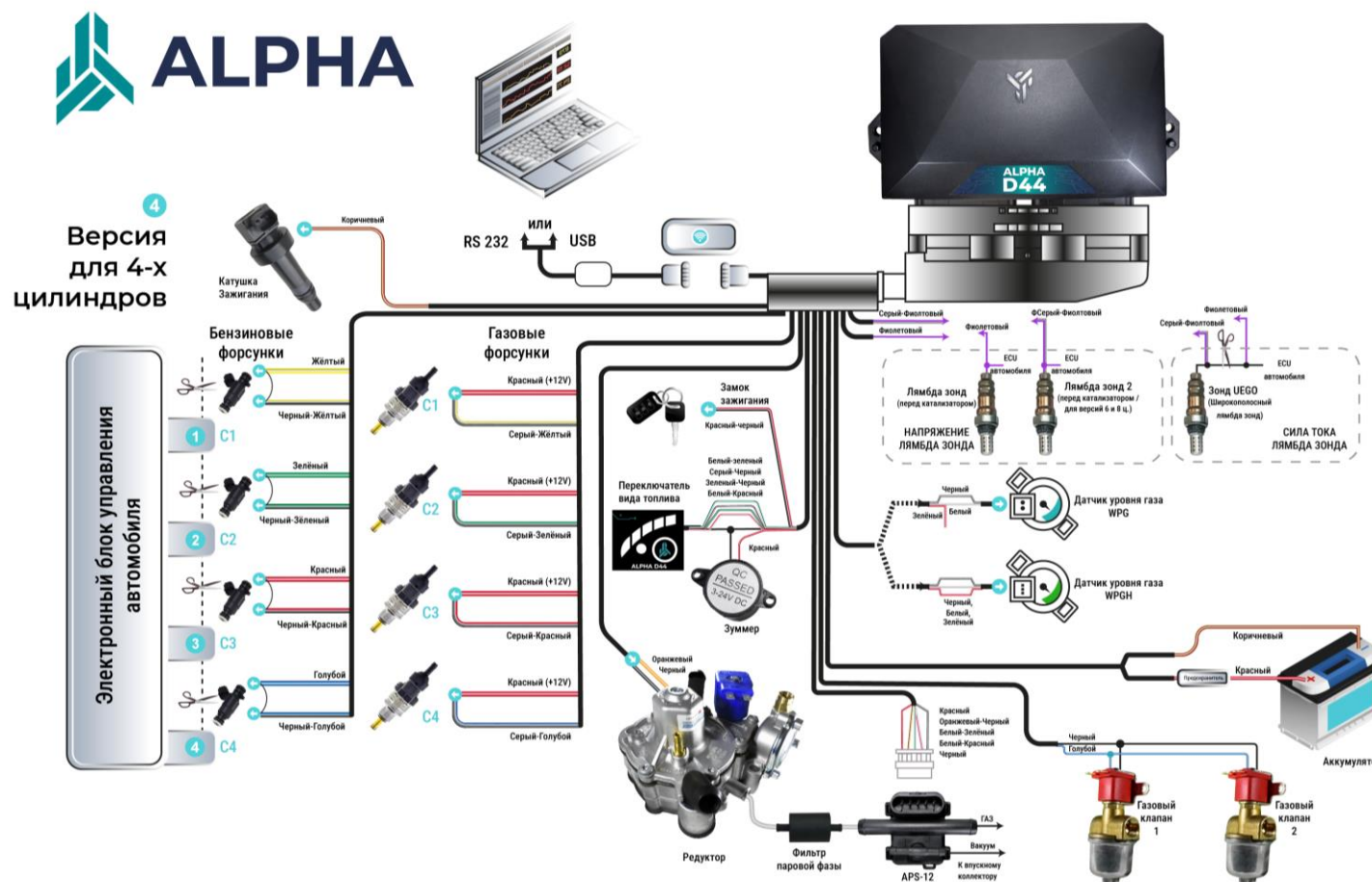
МОНТАЖНАЯ СХЕМА ALPHA D 44
